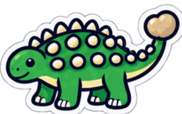
ankylosaurus
