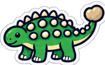
ankylosaurus
