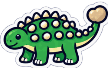
ankylosaurus
