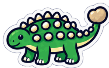
ankylosaurus
